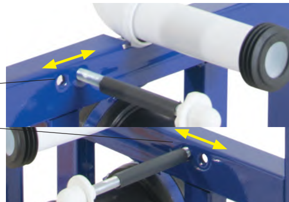
Ρυθμιζόμενες ντίζες
