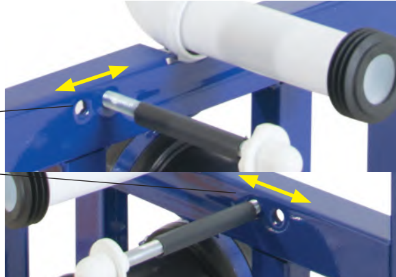
Ρυθμιζόμενες ντίζες
