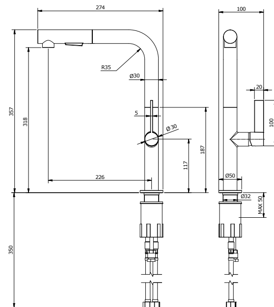
LEA με αποσπώμενο τηλέφωνο
