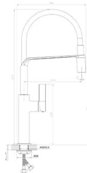
GAIA με περιστρεφόμενο ρουξούνι και αποσπώμενο ντους
