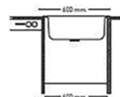
Ένθετος Νεροχύτης 60x50cm
