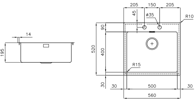
Νεροχύτης 56x52cm, Βάθος: 19,50cm, Πάχος: 1mm
