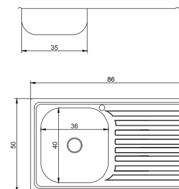
Ένθετος Νεροχύτης 86x50cm
