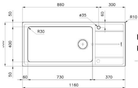
EVO Νεροχύτης 116x50cm, Βάθος: 17,5cm, Πάχος: 0,8mm
