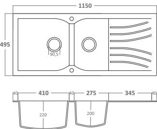
R-16 / 115x50cm, Βάθος: 22cm
