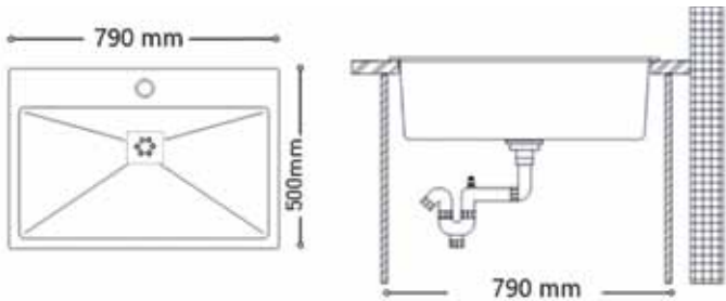
Ένθετος Χειροποίητος Νεροχύτης 79x50cm Με υποδοχή για Dispenser
