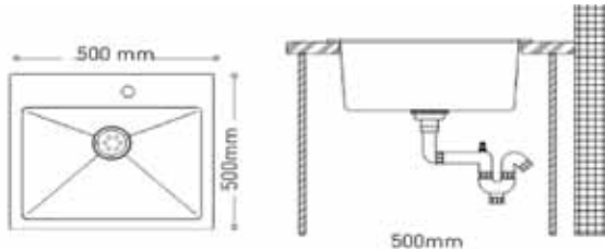
Ένθετος Χειροποίητος Νεροχύτης 50x50cm Με υποδοχή για Dispenser
