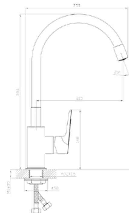
ANGELA White με ρυθμιζόμενο εύκαμπτο στόμιο σιλικόνης με 360° περιστροφή
