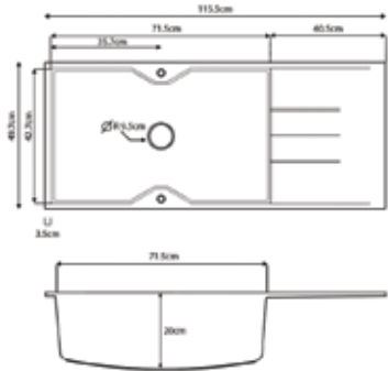
Νεροχύτης Q-16, 116x50cm, Βάθος: 20cm
