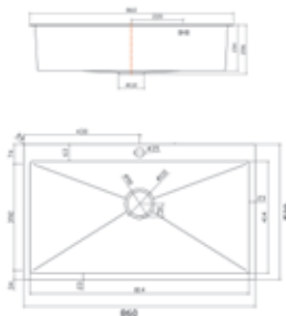
Ένθετος Νεροχύτης 86x50cm Black
