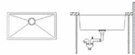
Υποκαθήμενος Χειροποίητος Νεροχύτης 79x50cm Copper
