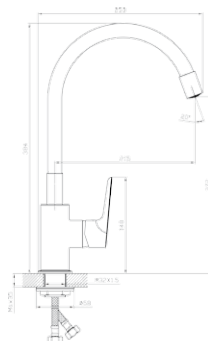
ANGELA Cappuccino με ρυθμιζόμενο εύκαμπτο στόμιο σιλικόνης με 360° περιστροφή
