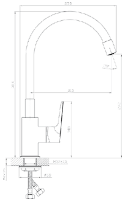
ANGELA Black με ρυθμιζόμενο εύκαμπτο στόμιο σιλικόνης με 360° περιστροφή
