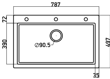
Νεροχύτης Q-81, 79x50cm, Βάθος: 20cm
