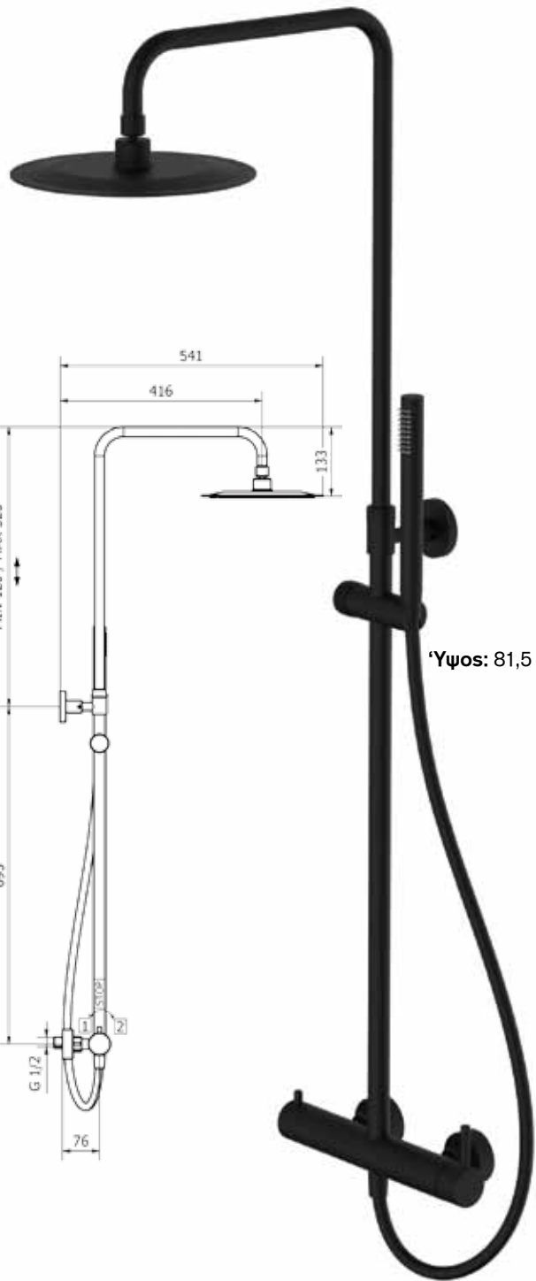
Κολώνα ντους με τηλέφωνο, σπιράλι και κεφαλή Ø25cm Inox, βέργα ρυθμιζόμενη καθ' ύψος
