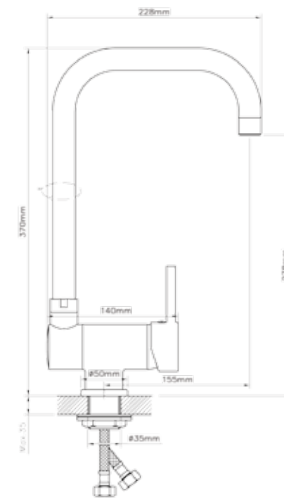
ERI με ανακλινόμενο και περιστρεφόμενο ρουξούνι 360°
