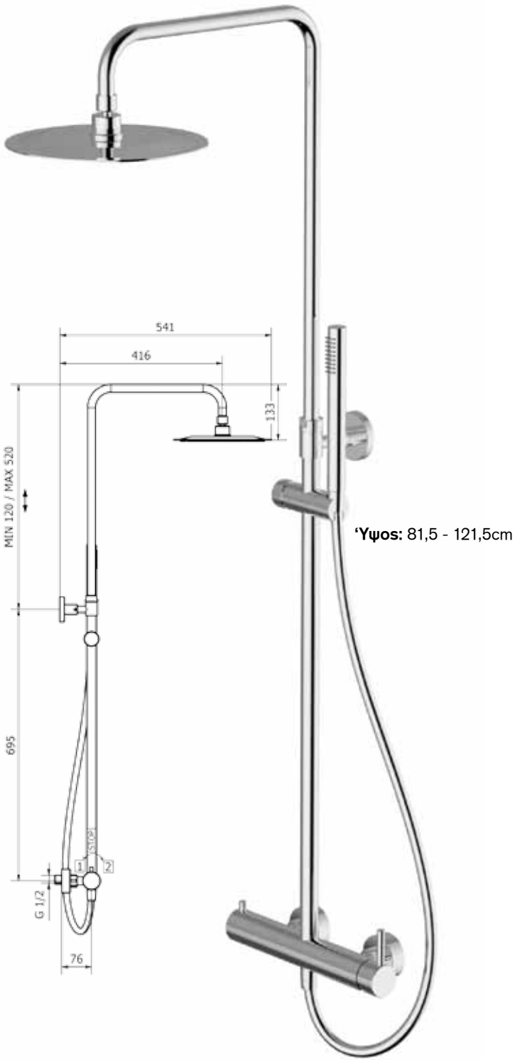
Κολώνα ντους με τηλέφωνο, σπирάη και κεφαλή Ø25cm Inox, βέργα ρυθμιζόμενη καθ' ύψος
