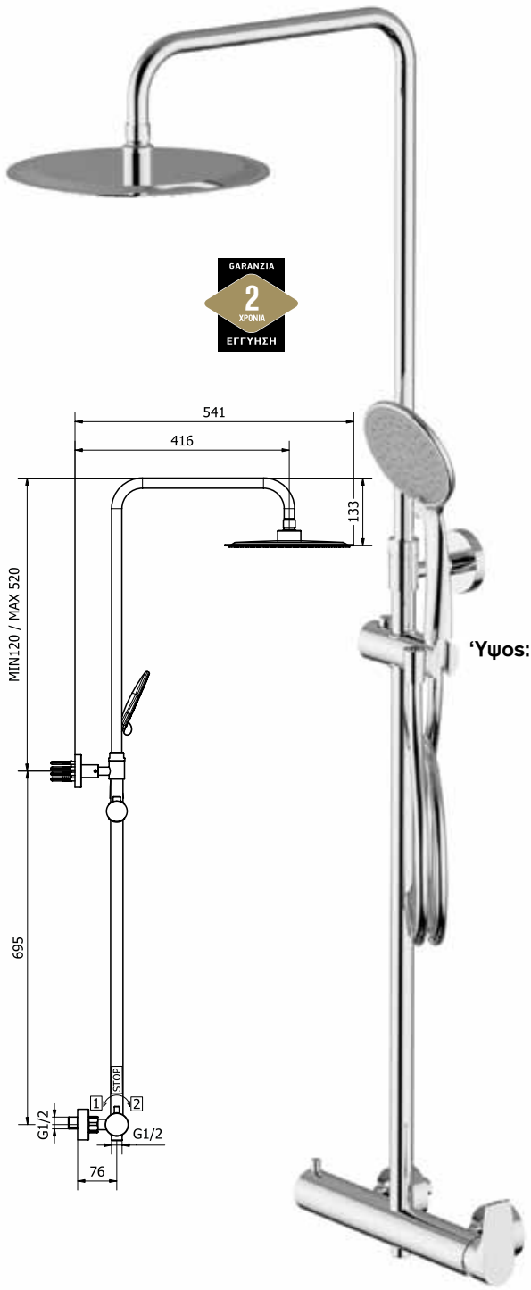
Κοιλώνα ντους με μπαταρία, τηλέφωνο ντους 3 ροών, σπιράλ 150cm PVC, κεφαλή ντους Inox στρογγυλή Ø25cm, βέργα ρυθμιζόμενη καθ' ύψος
